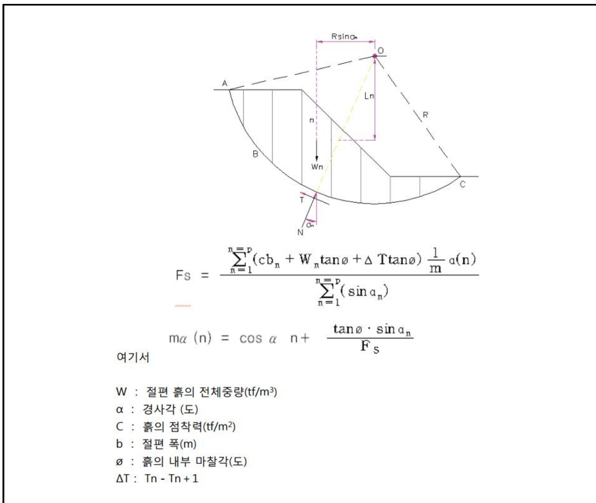
【그림 64.7】 Bishop의 안전율 계산식
